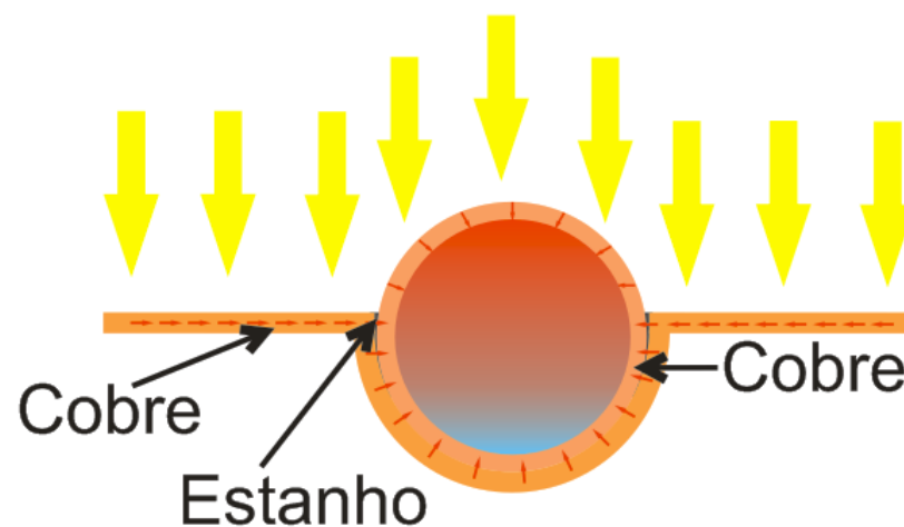
Coletor Aquesol
