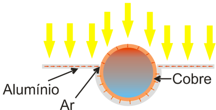
Coletor Comum
